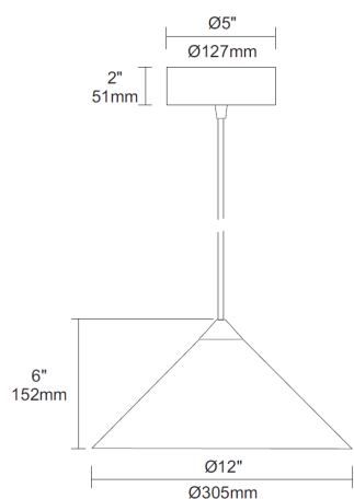
FRONT VIEW VUE DE FACE
