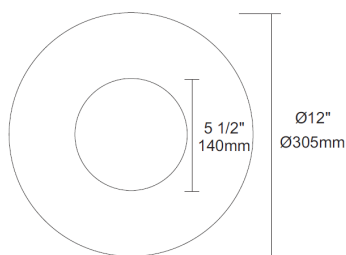
BOTTOM VIEW VUE DE DESSOUS
