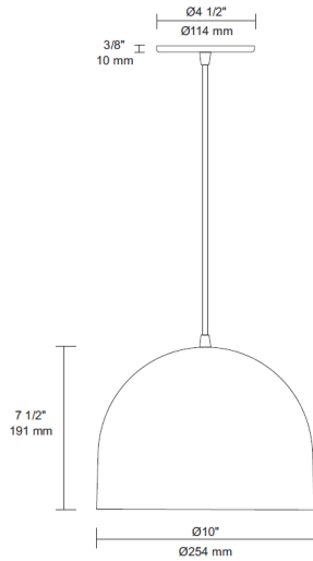
FRONT VIEW VUE DE FACE
