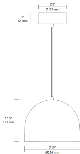
FRONT VIEW VUE DE FACE
