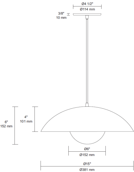
FRONT VIEW VUE DE FACE
