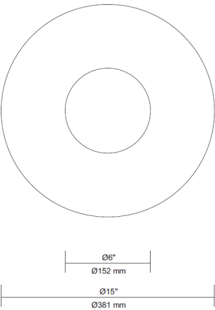
BOTTOM VIEW VUE DE DESSOUS
